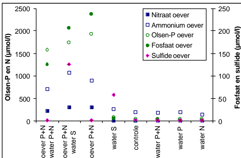
Figuur 4.38 Het effect van de verschillende behandelingen op de concentraties nutriënten en sulfide in de oever.
